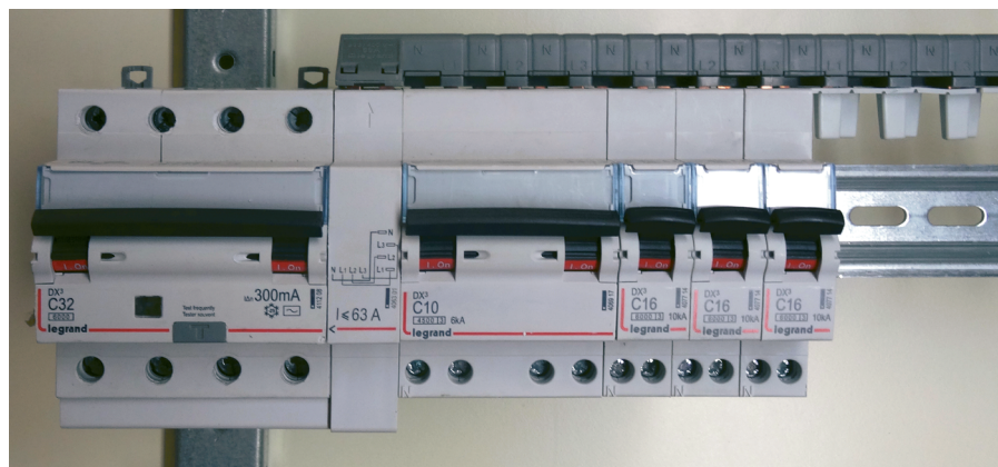
Groupe triphasé avec disjoncteur en tête et répartition par peigne tétrapolaire HX 3 optimisé
