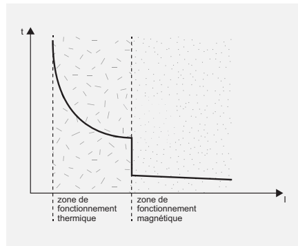
Zones de déclenchement d'un disjoncteur magnétothermique
