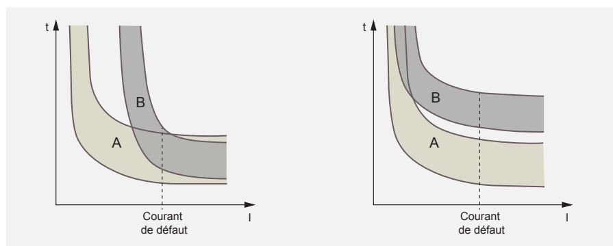
Sélectivité partielle entre deux DDR non retardés de sensibilités différentes : mauvaise sélectivité
