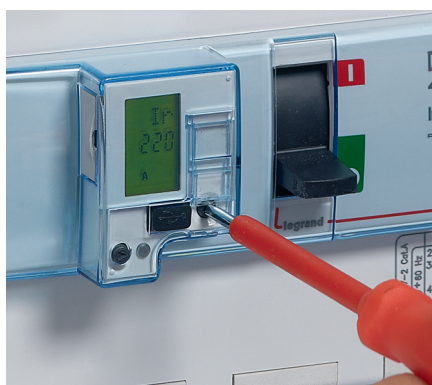
Réglage de la sélectivité dynamique sur DPX 3
