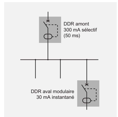
Sélectivité totale à deux niveaux
