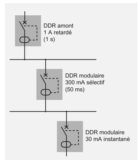
Sélectivité totale à deux niveaux
