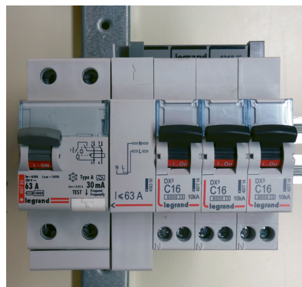
Groupe monophasé avec interrupteur différentiel en tête et répartition par peigne universel HX 3 optimisé
