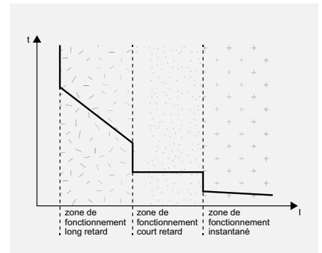
Zones de déclenchement d'un disjoncteur électronique
